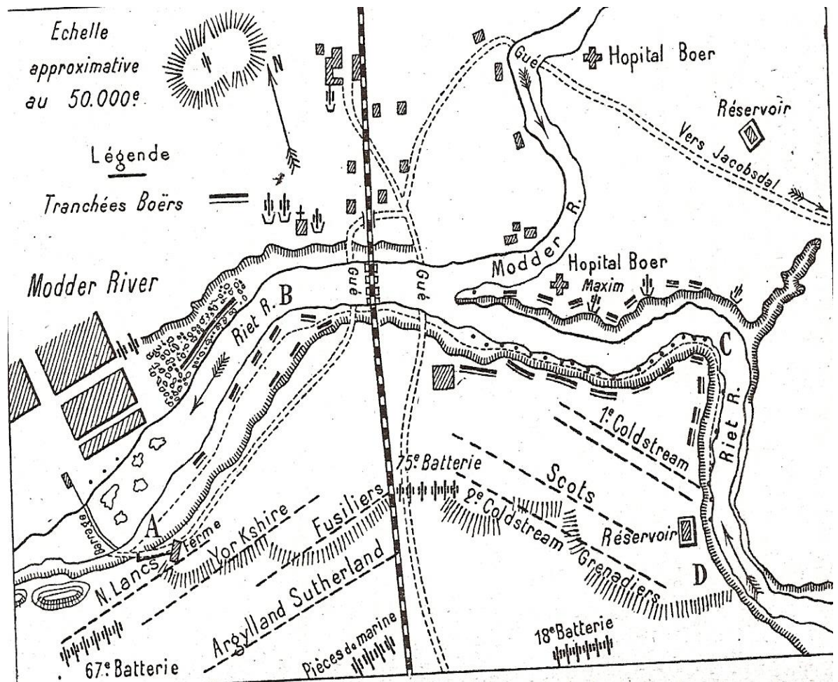
Croquis del Capitan Gilbert. Los ingleses tienen 9.000 hombres y 22 cañones. Los federados tienen aproximadamente 7.000 hombres y 10 cañones. (Croquis Gilbert)
